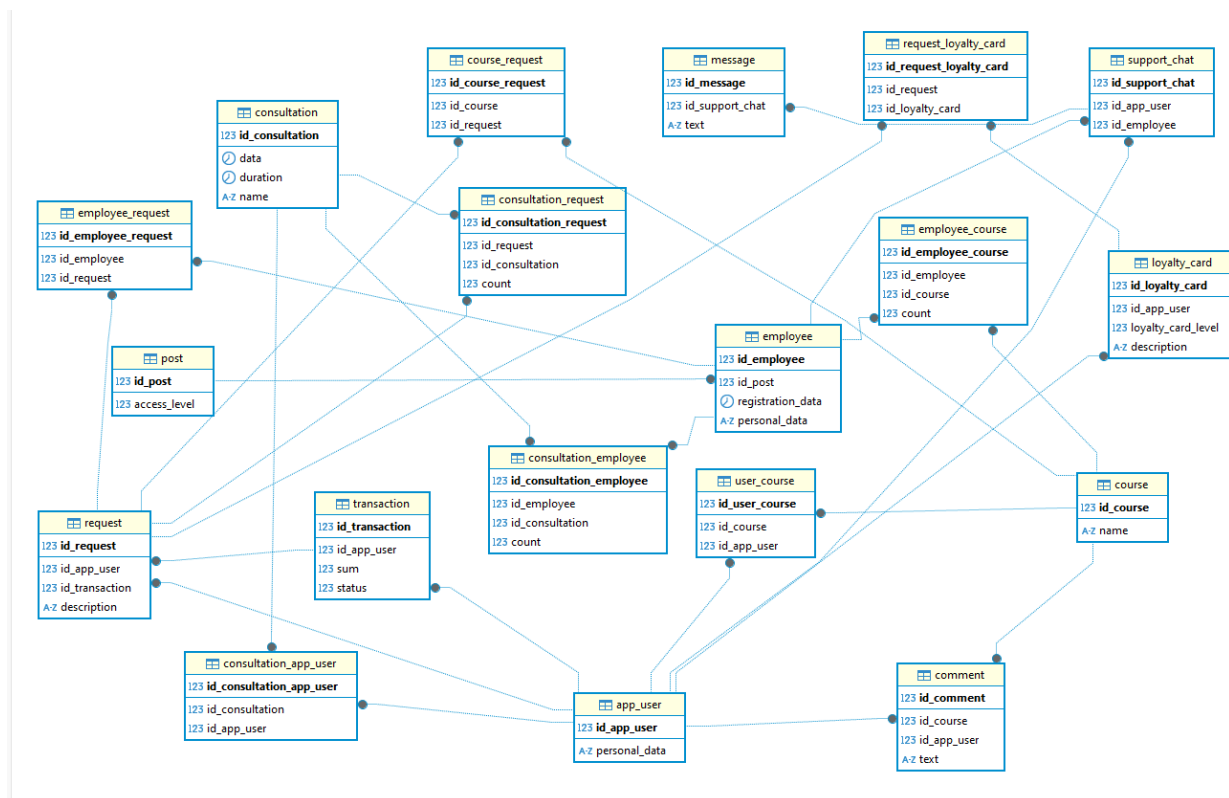
Рисунок 4 – Отображение итоговой базы данных в графическом виде
